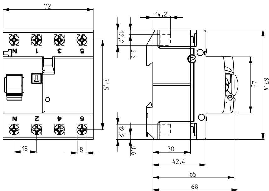
G/KV - Reset (100 & 125A)
